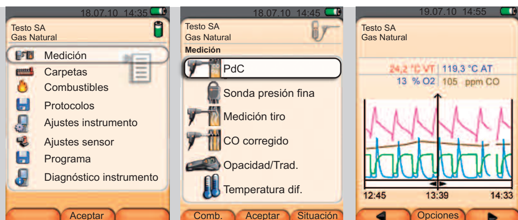
Menú principal - selección de funciones
