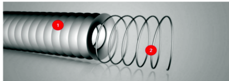
Tubería fabricada con tejido de PVC con espiral de refuerzo de alambre cincado
