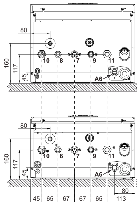
Vista inferior
