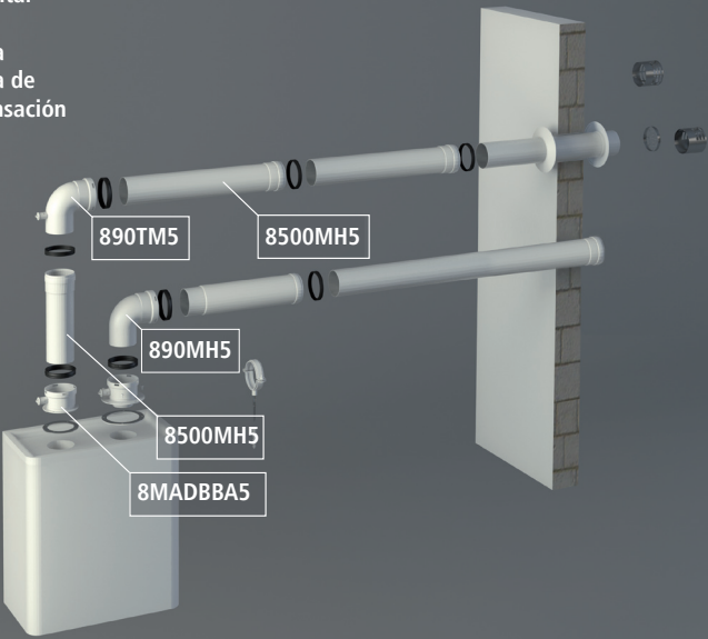
Esquema salida Horizontal
