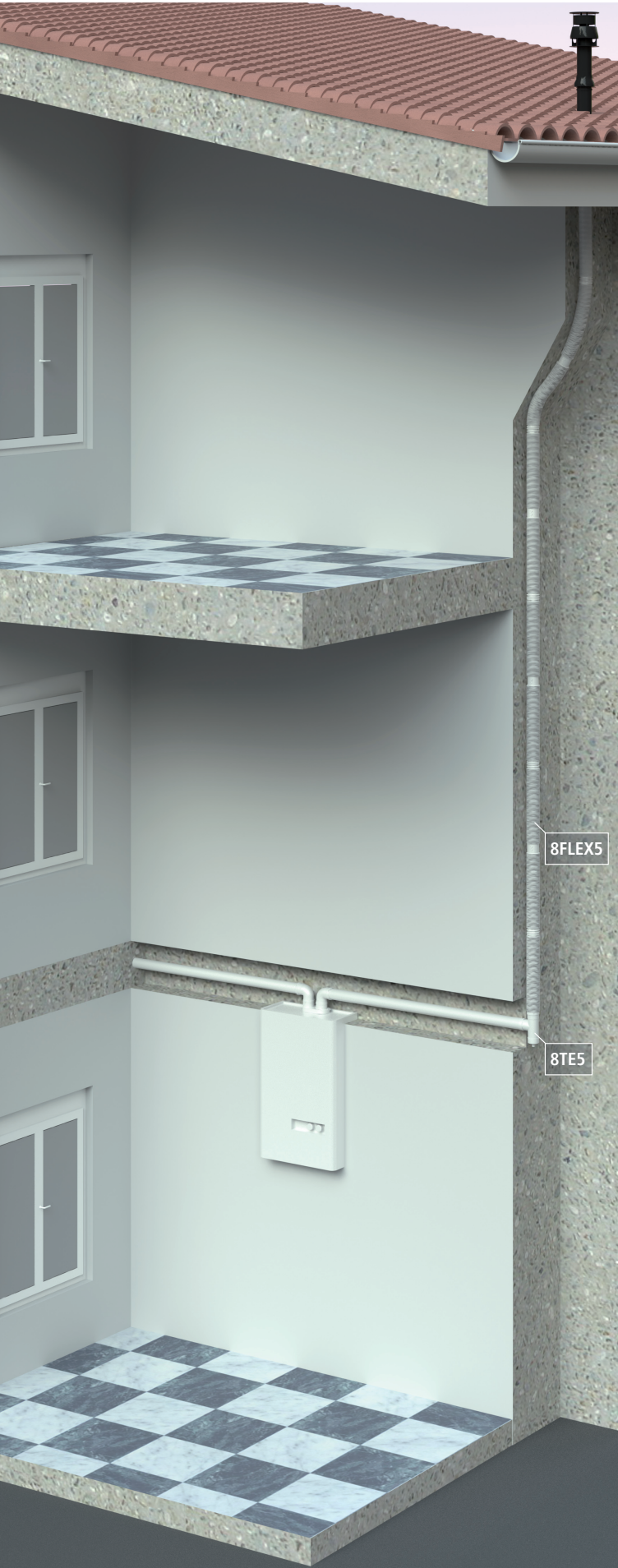
Esquema Montaje Instalación Tubo Flexible Caldera Estanca Condensación
