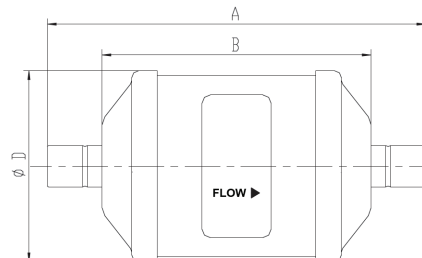
Conexión Soldar
