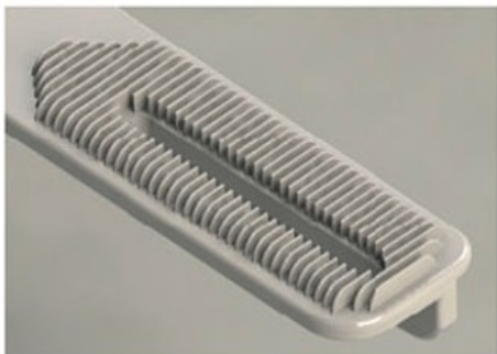
Detalle Silents-Bloks integrados en el mismo molde termoplástico.
