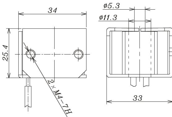
Dibujo 1: FQA-55001, -55002, -55003
