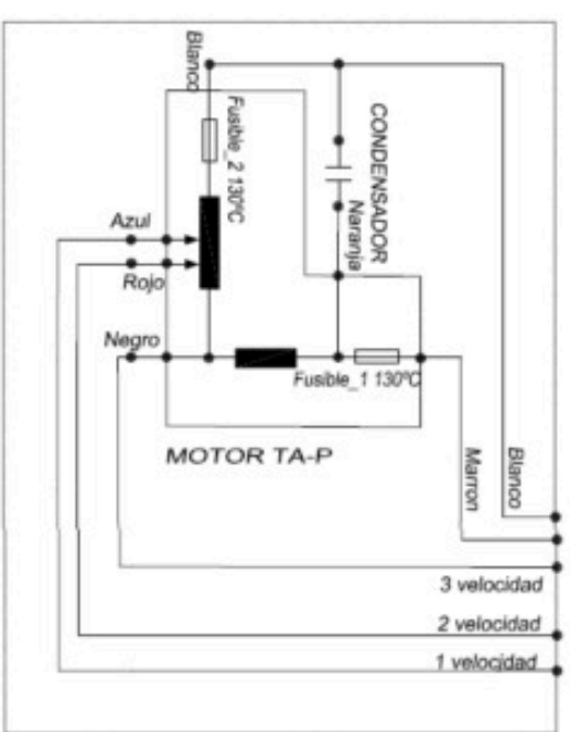
Conexión Motor
